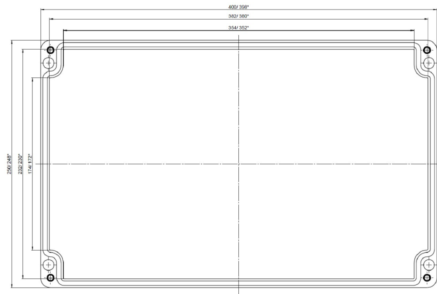
Deckel / Lid
